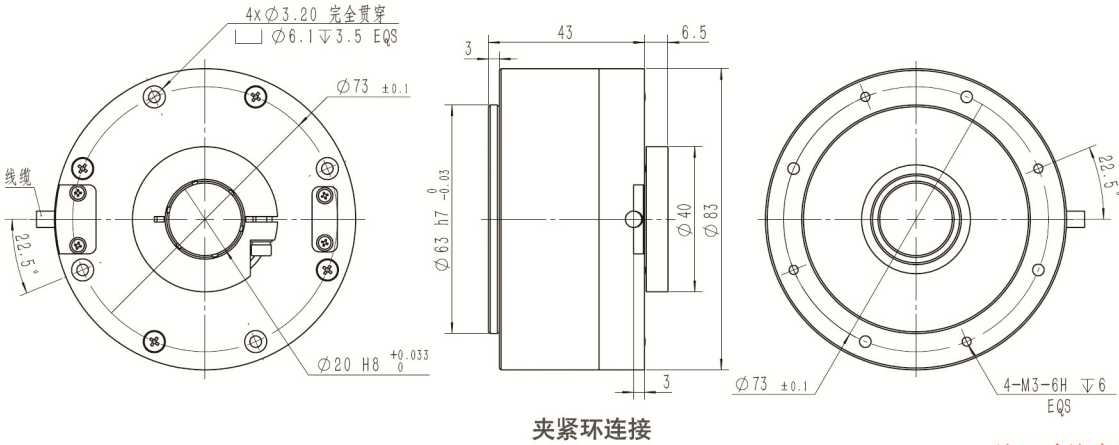
夹紧环连接
