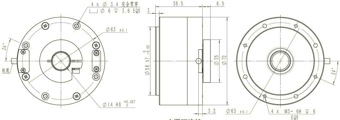
夹紧环连接
