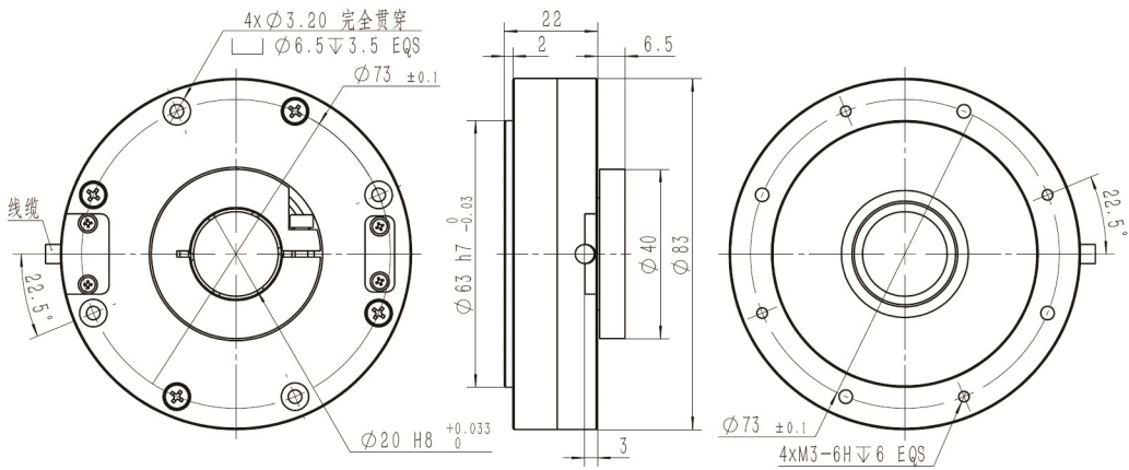
夹紧环连接
