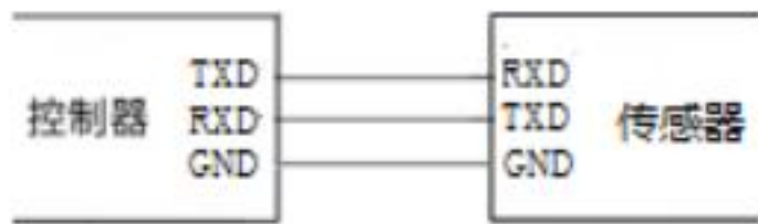
图 5 RS232 电气连接图
