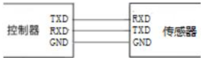
图 5 RS232 电气连接图
