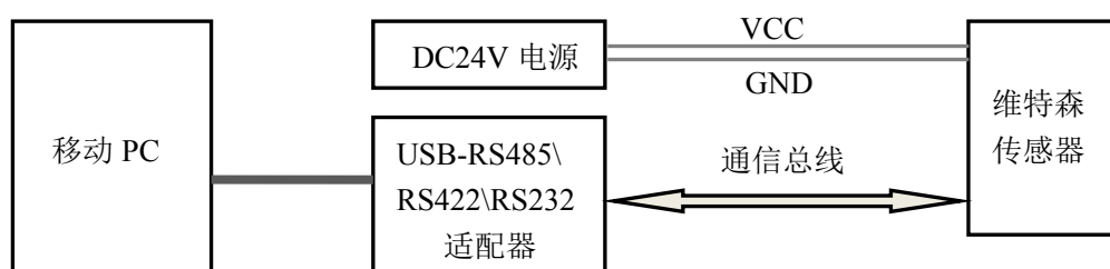
图 7 传感器配置电气连接图
